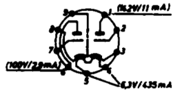
ECC 85
